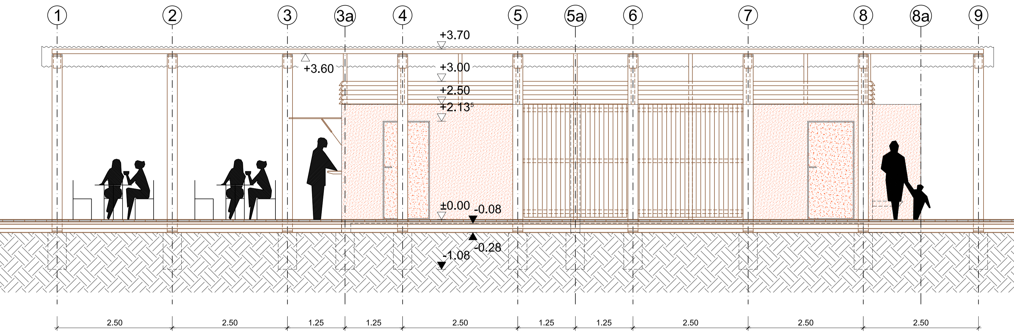
ANSICHT OST
