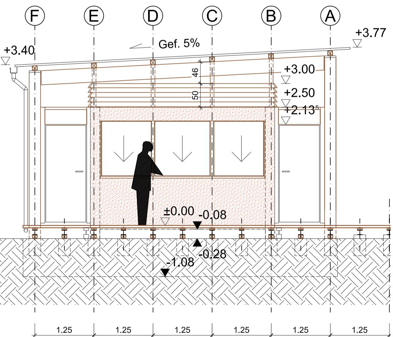
ANSICHT SÜD
