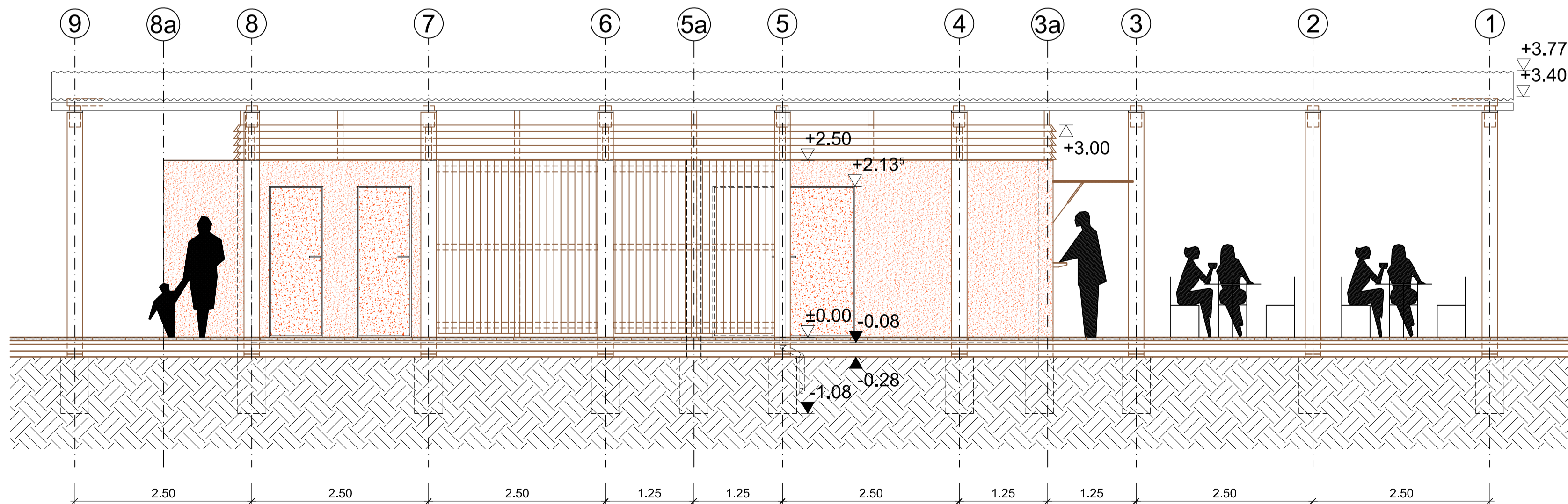
ANSICHT WEST
